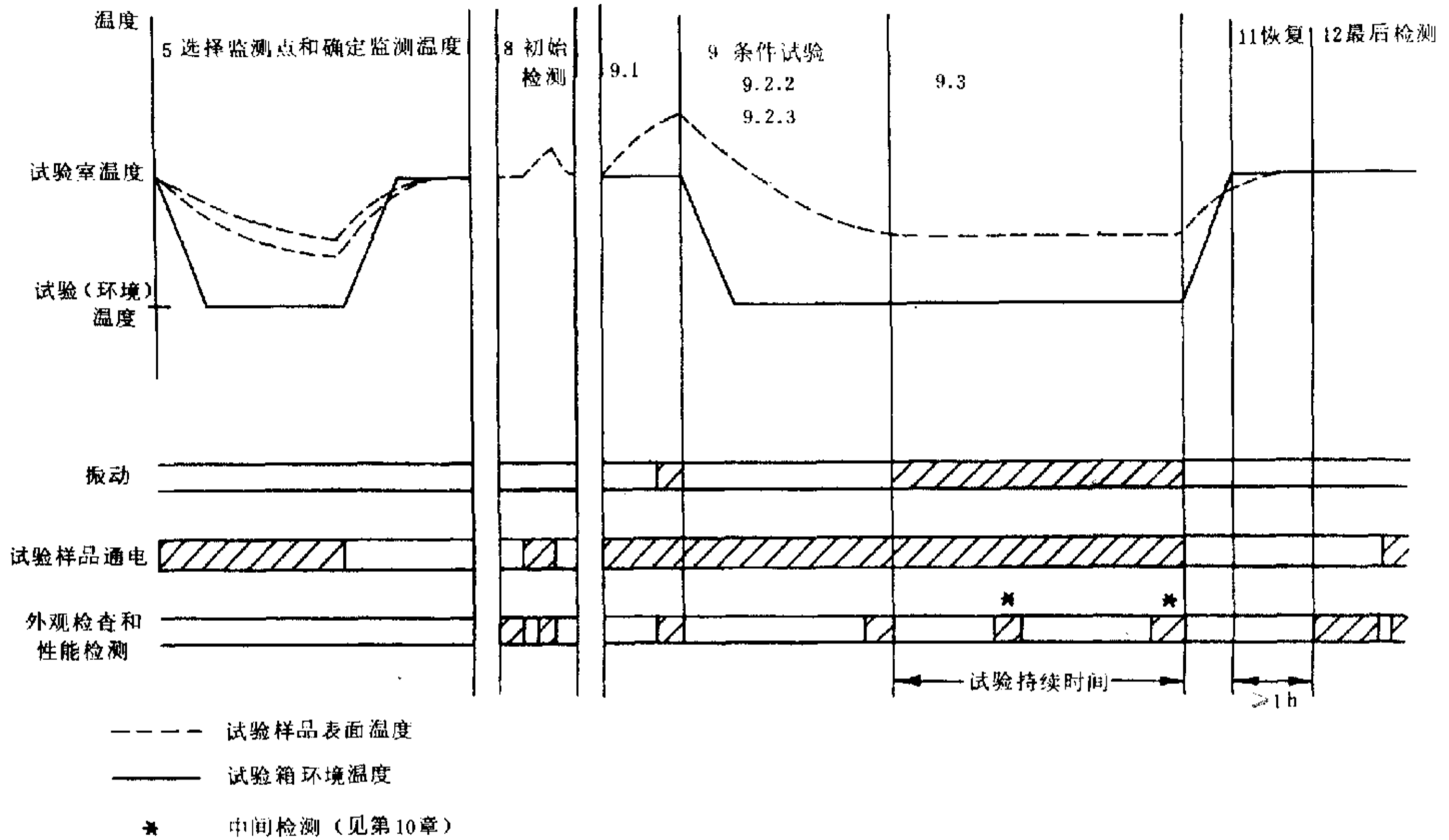
图 2 散热试验样品试验曲线图
